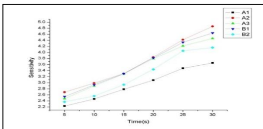
ภาพที่ 5 การตอบสนองต่อแก๊ส Ethanol ของ โครงสร้างนาโน CuO
